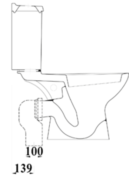
Venezia WC P
